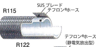
■ ホース構造図
