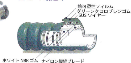
■ ホース構造図
